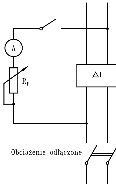
Rys. 5. Sprawdzanie działania urządzenia ochronnego różnicowoprądowego metodą 2
